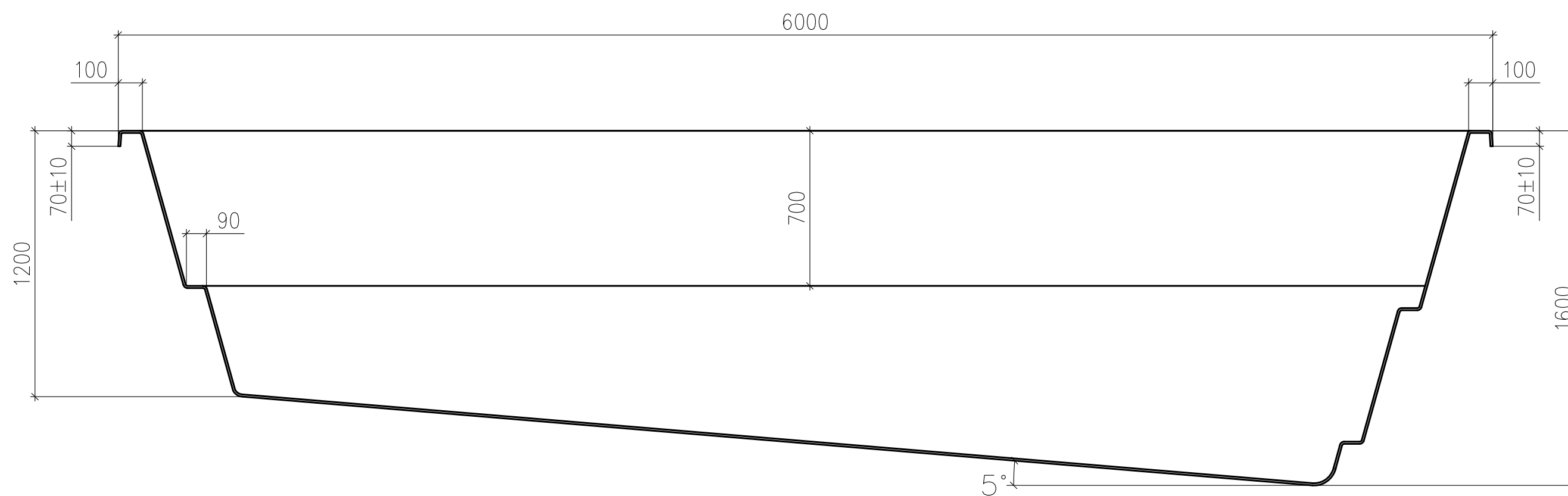
Разрез 1 – 1
